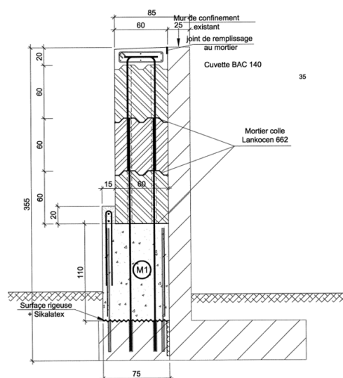
COFFRAGE TYPE MUR POIDS BAC 140
